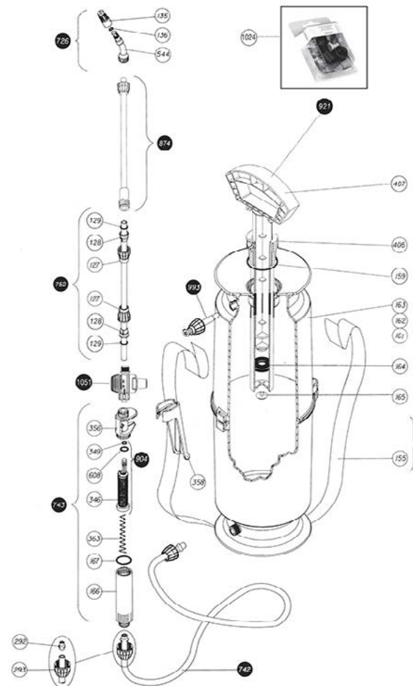
COUDE HERBICIDES FAIBLE VOLUME code 8.34.60.935
